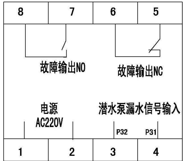
面板上 绿灯为电源指示；红灯为泄漏故障指示。 潜水泵漏水保护器接线端子图
